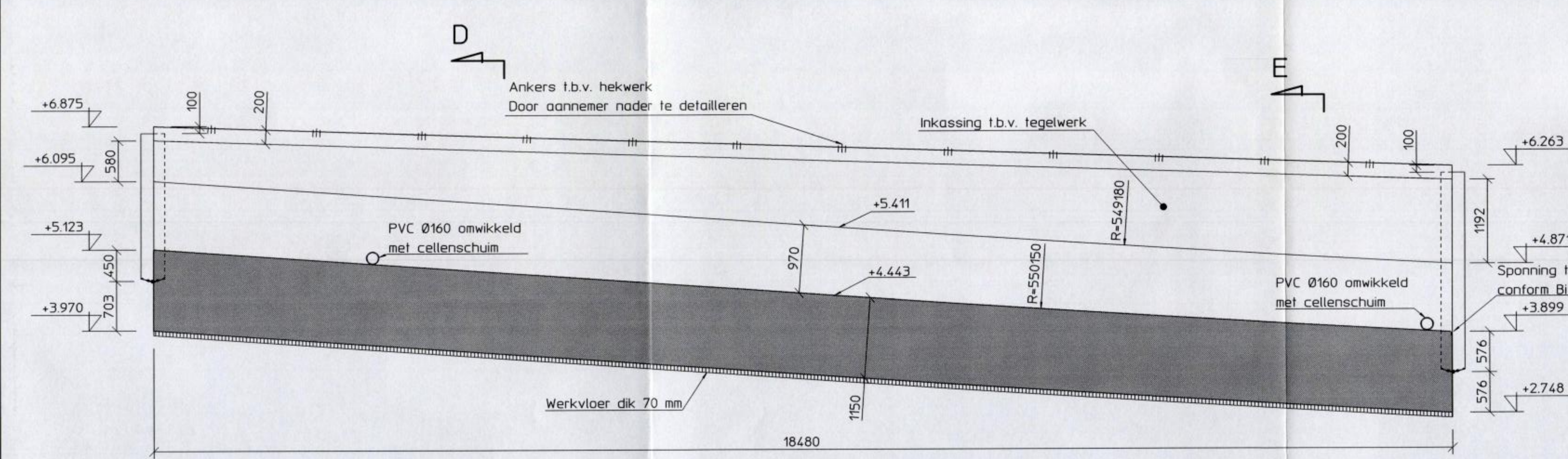
Doorsnede B schaal 150
