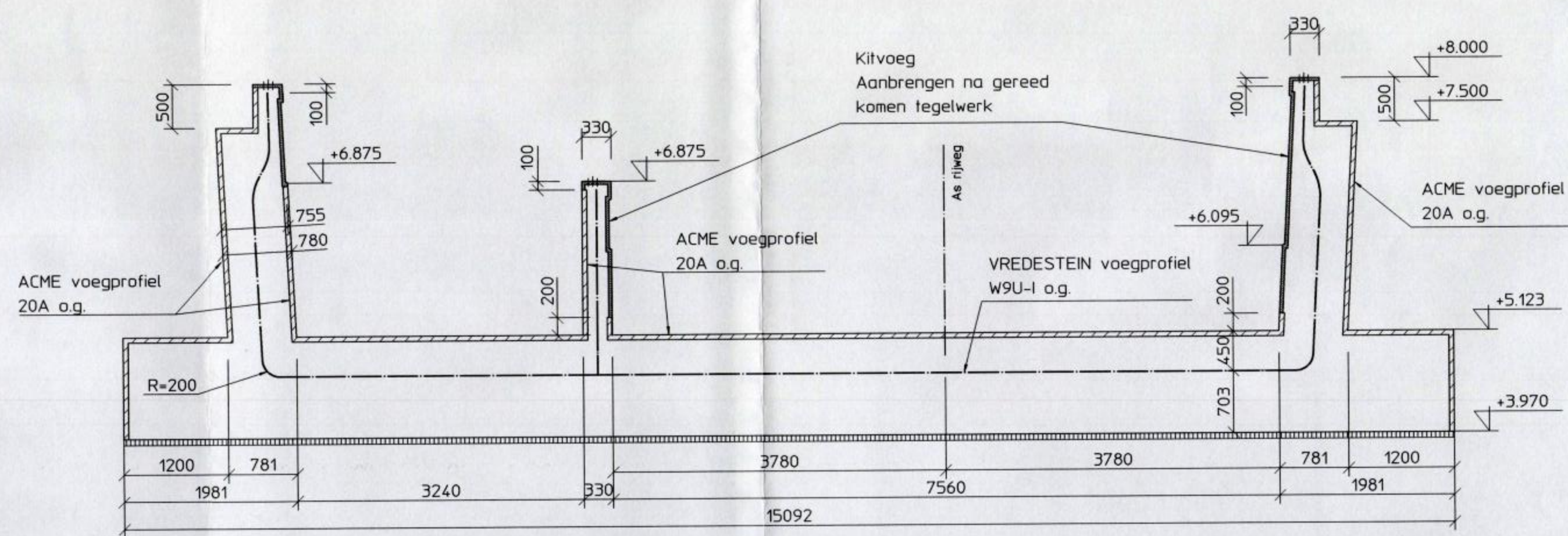
Aanzicht G schaal 150
