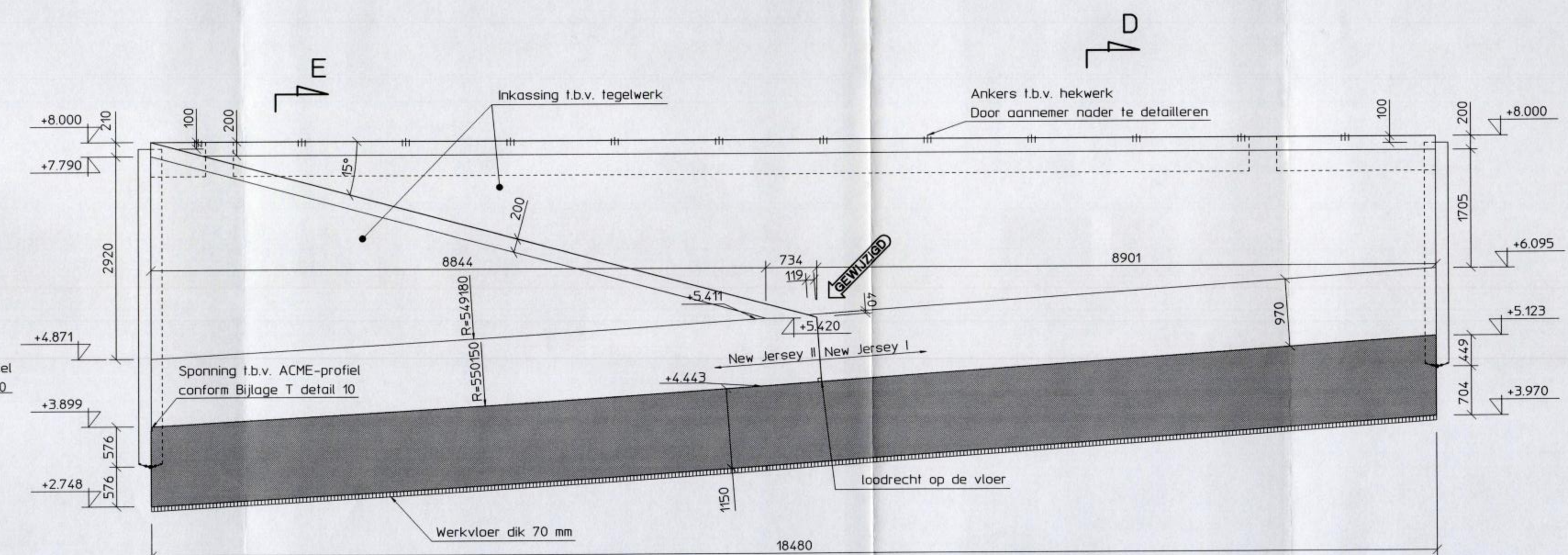
Doorsnede C schaal 150
