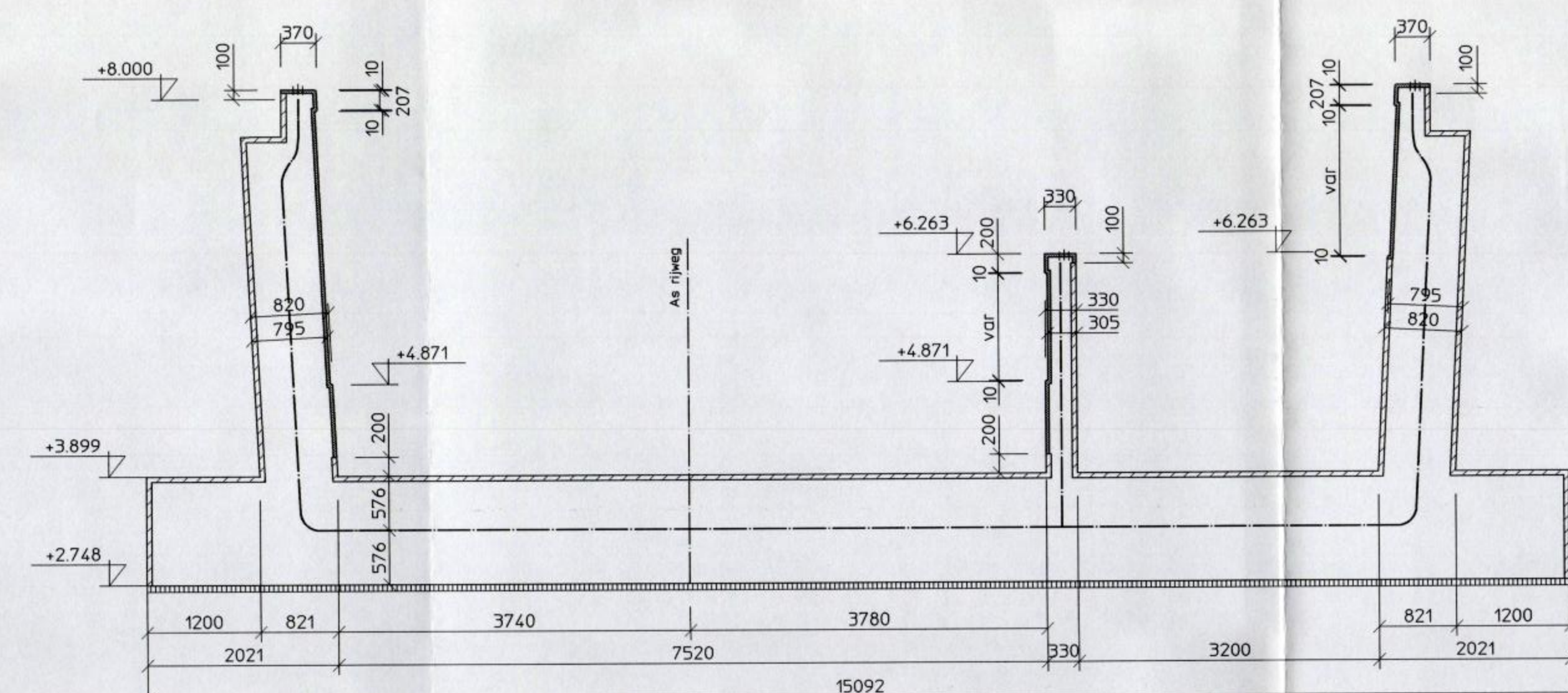
Aanzicht F schaal 150
