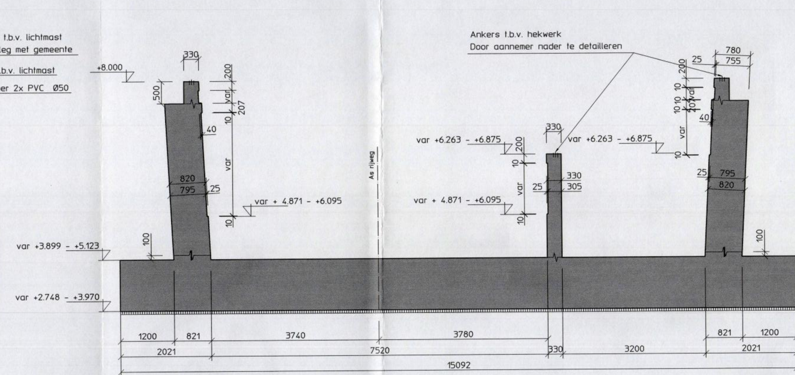
Doorsnede E schaal 150
